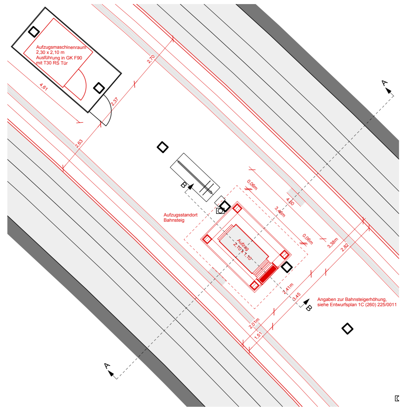
Grundriss Bahnsteige Ebene, M 1:100
