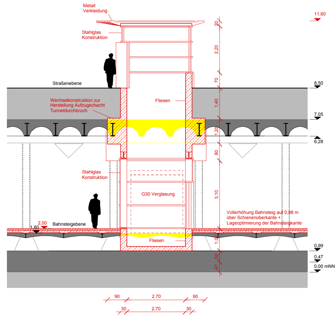
Schnitt B-B, M 1:100
