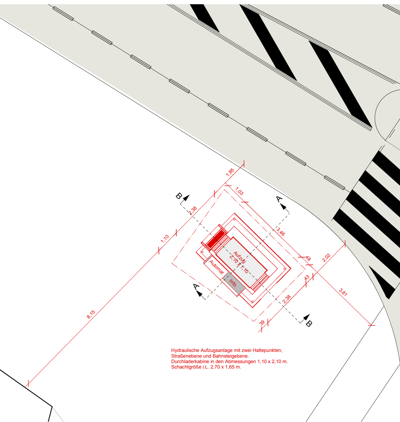
Grundriss Straßenebene, M 1:100
